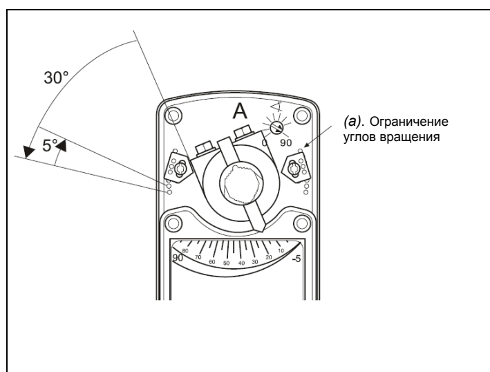
Рисунок 6: Ограничение диапазона углов вращения
