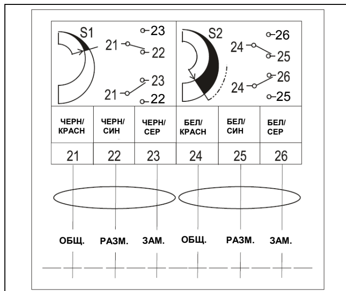
Рисунок 9: Схема электрического подключения концевых выключателей
